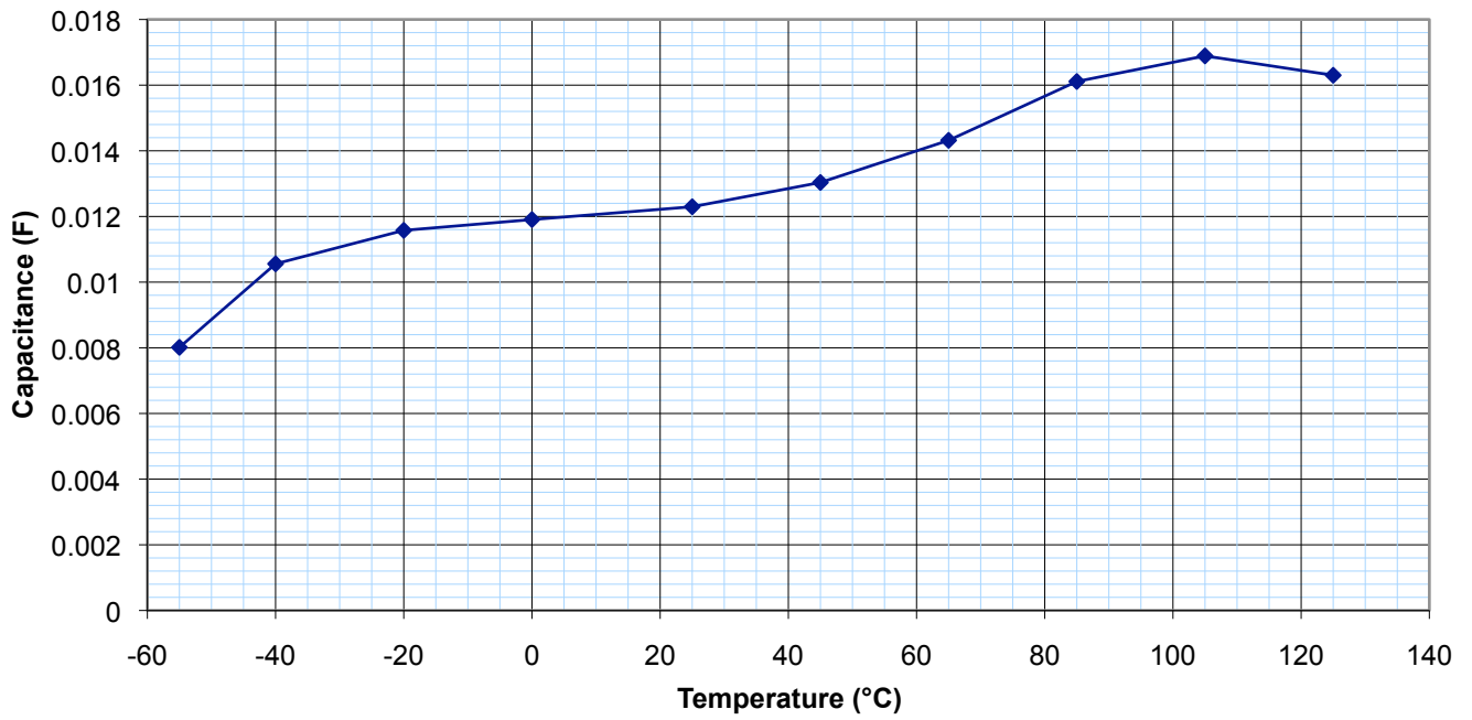
THQ1035123 (120Hz)
