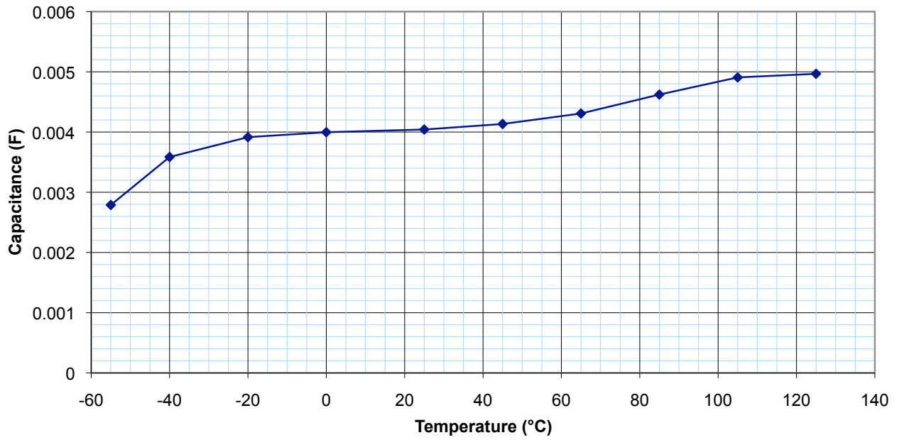
THQ1063402 (120Hz)
