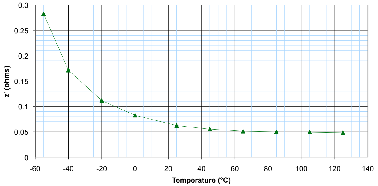
THQ1063402 (1kHz)
