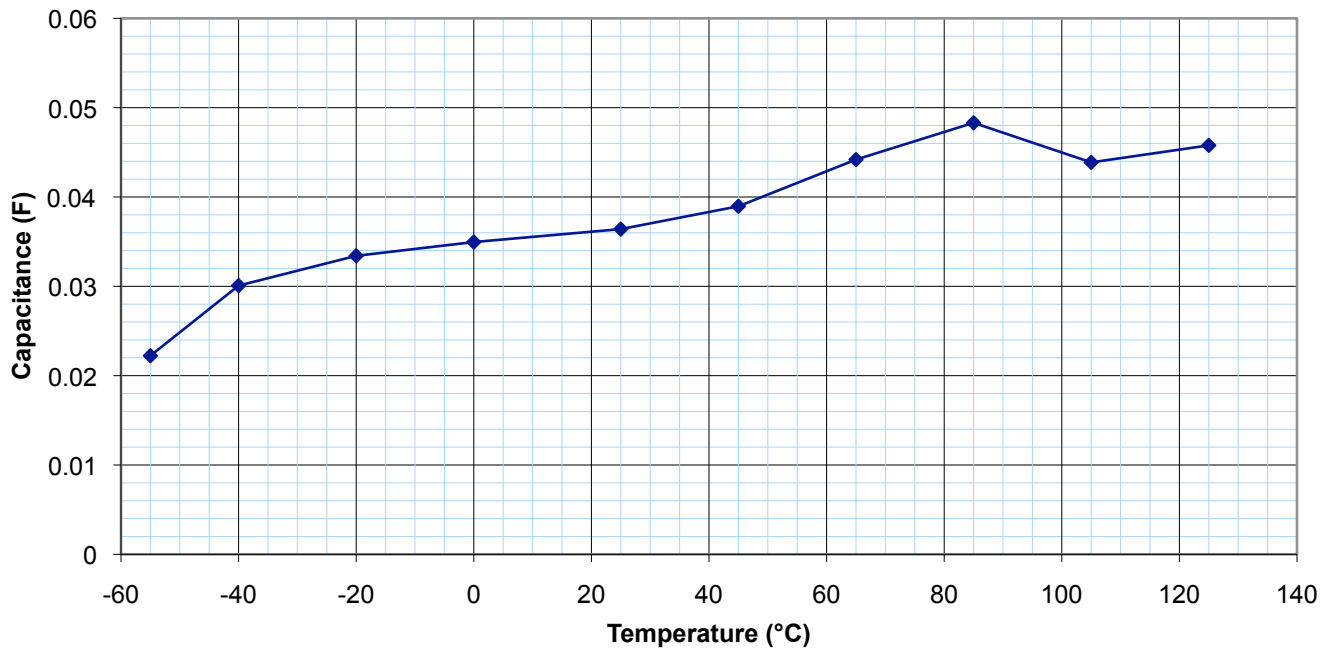
THQ3035363 (120Hz)
