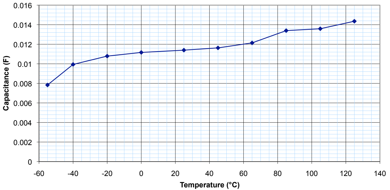
THQ3063123 (120Hz)
