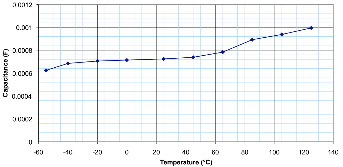
THQA2060871 (120Hz)
