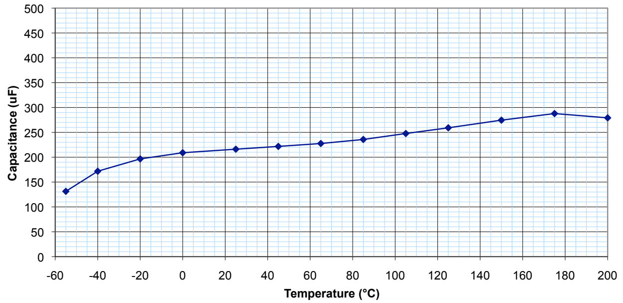
THQA2125211HT (120Hz)
