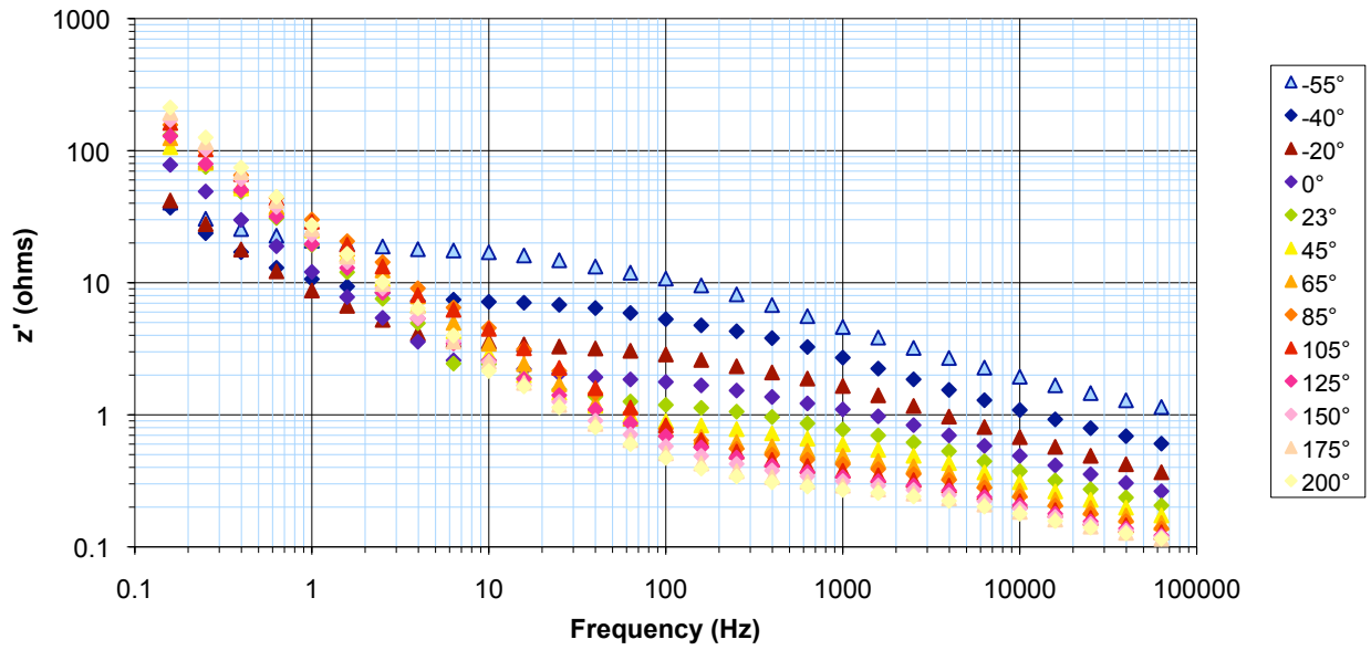
THQA2125211HT
