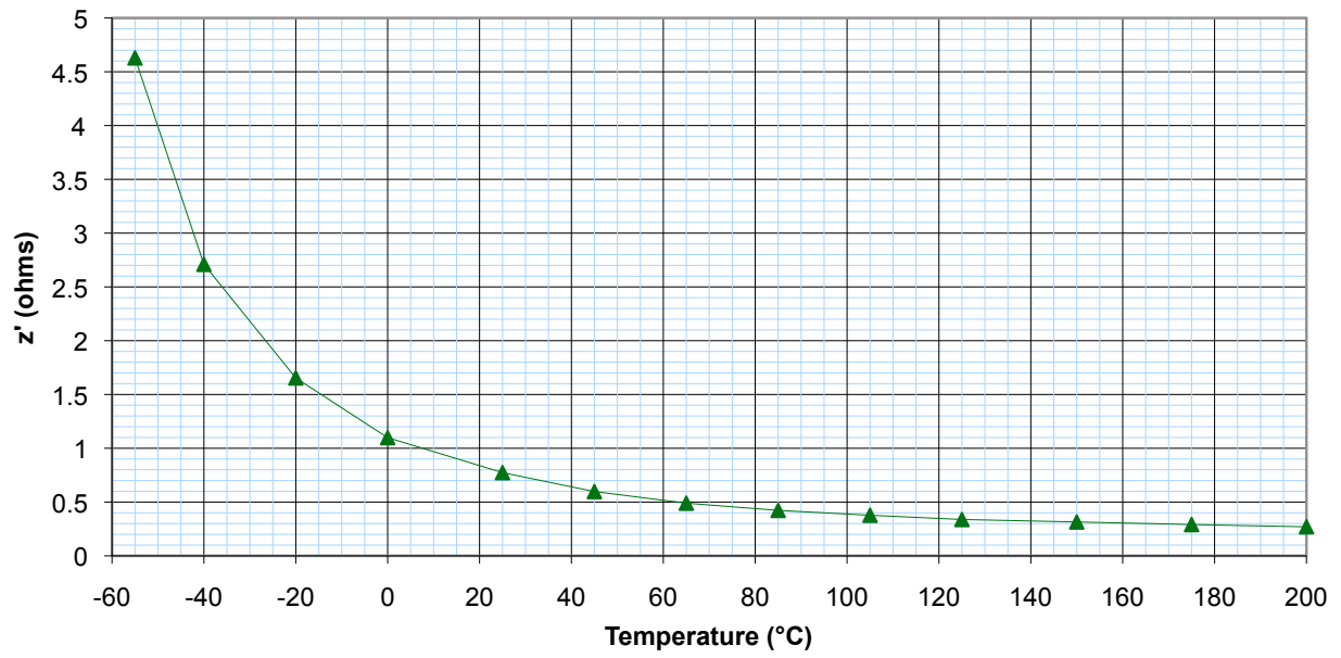
THQA2125211HT (1kHz)
