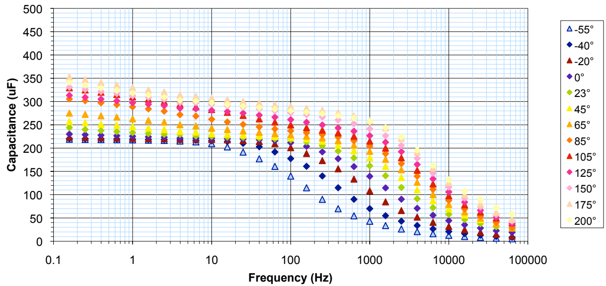
THQA2125211HT
